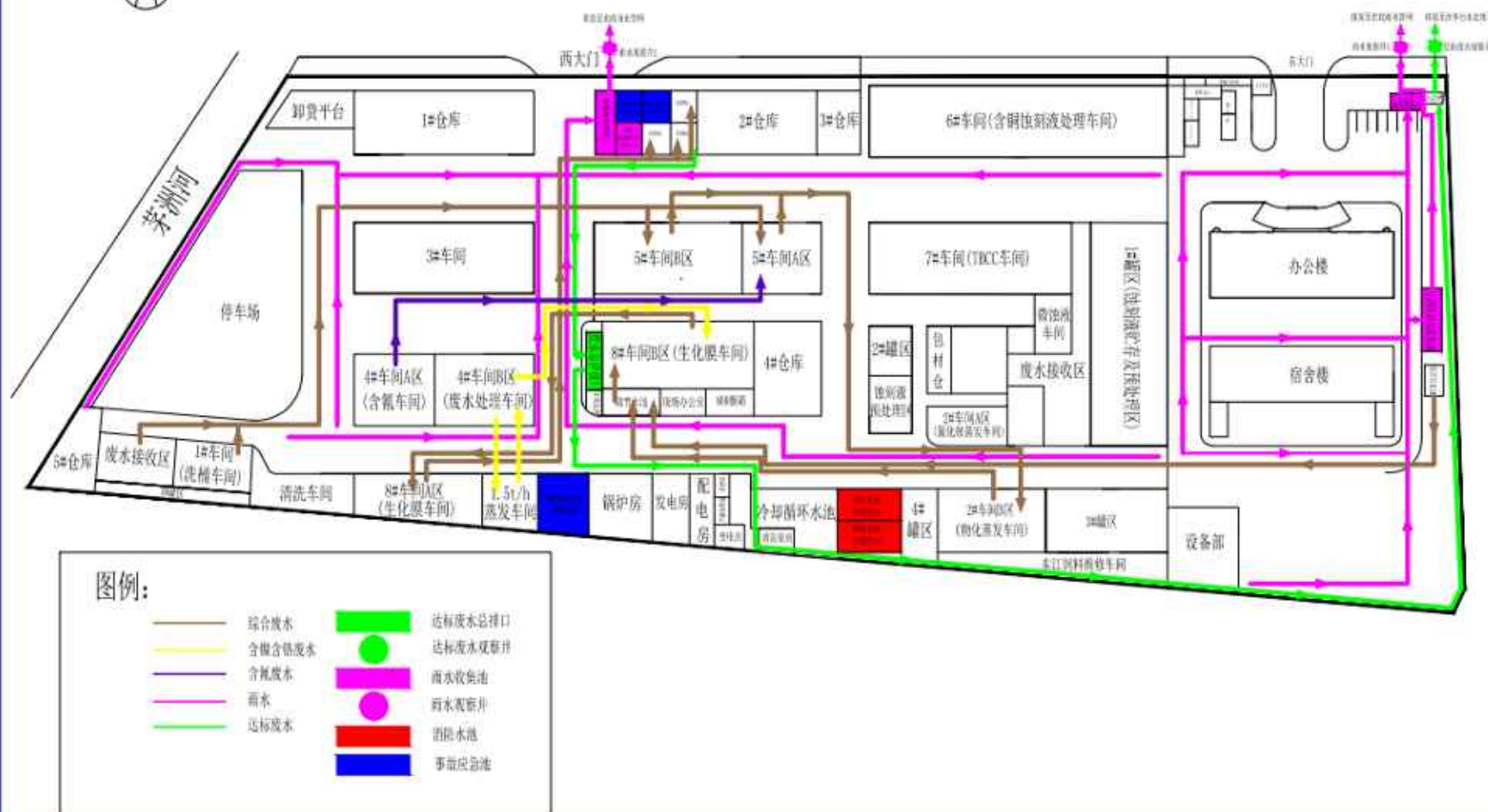
深圳市宝安东江环保技术有限公司雨水、污水管网及应急设施分布图
