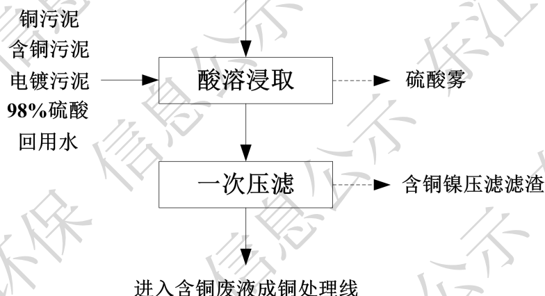
图 3.3-6 含铜废液综合酸溶压滤预处理线工艺流程和产物环节图
