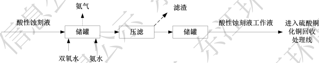
图 2.3-10 硫酸铜预处理线工艺流程及产污环节图
