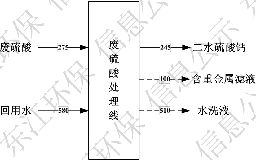
图 3.3-44 废硫酸处理线水平衡图 单位:m³/a
