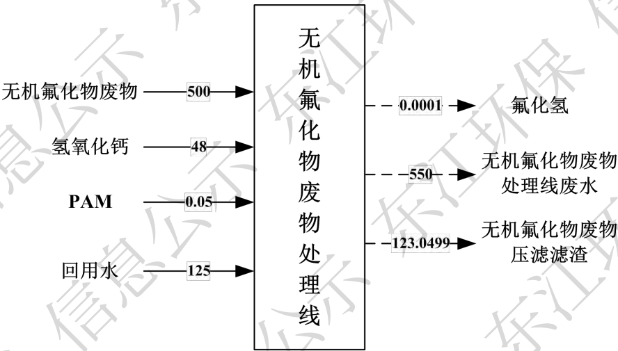
图 3.3-45 无机氟化物废物处理线物料平衡图 单位:t/a
